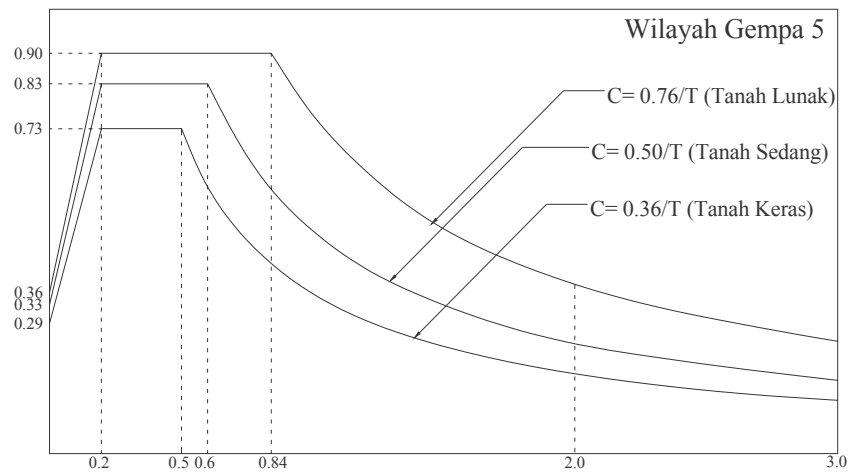
Gambar 2.8 Spektrum respon Gempa Zona 5
