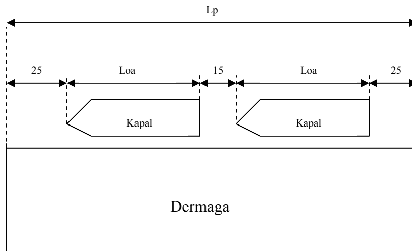
Gambar 2.4 Panjang Dermaga
